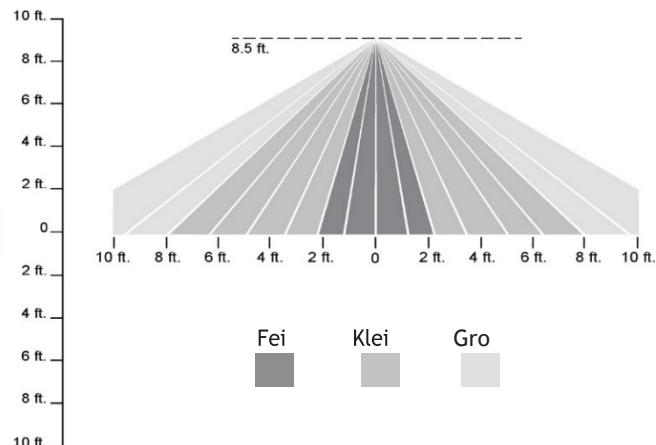
Seitenansicht
