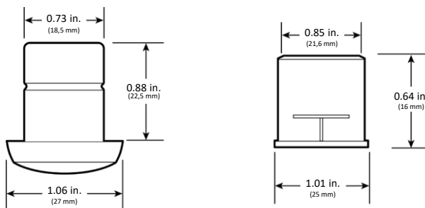
Mikrosensor (SU-5E)
